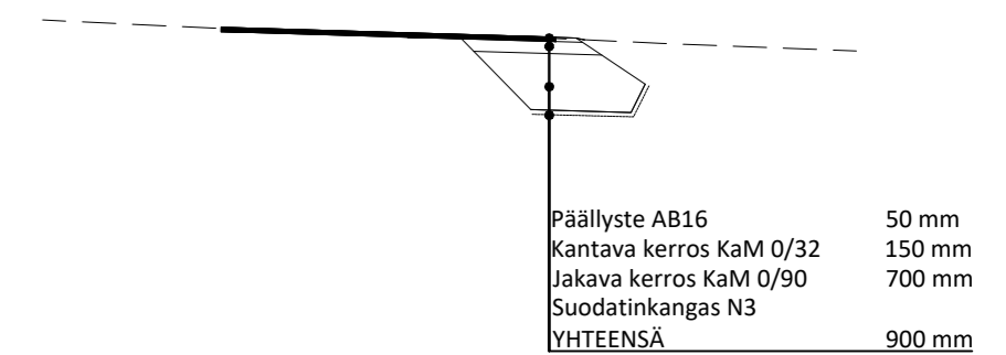
Mäki-Hovintien, Koulutien ja Pappilanraitin pysäköintialueiden levennysrakenne
