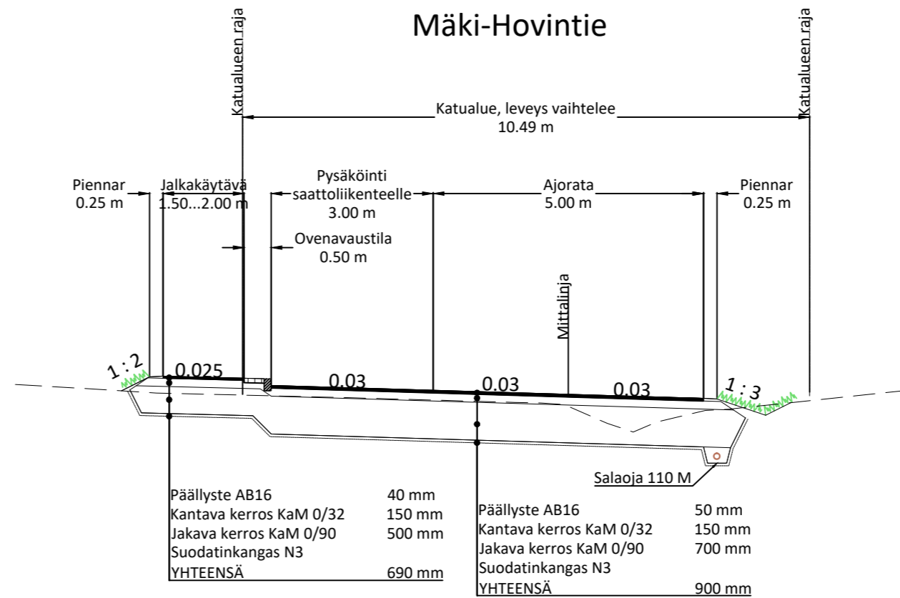
Mäki-Hovintien, Koulutien ja Pappilanraitin pysäköintialueiden levennysrakenne
